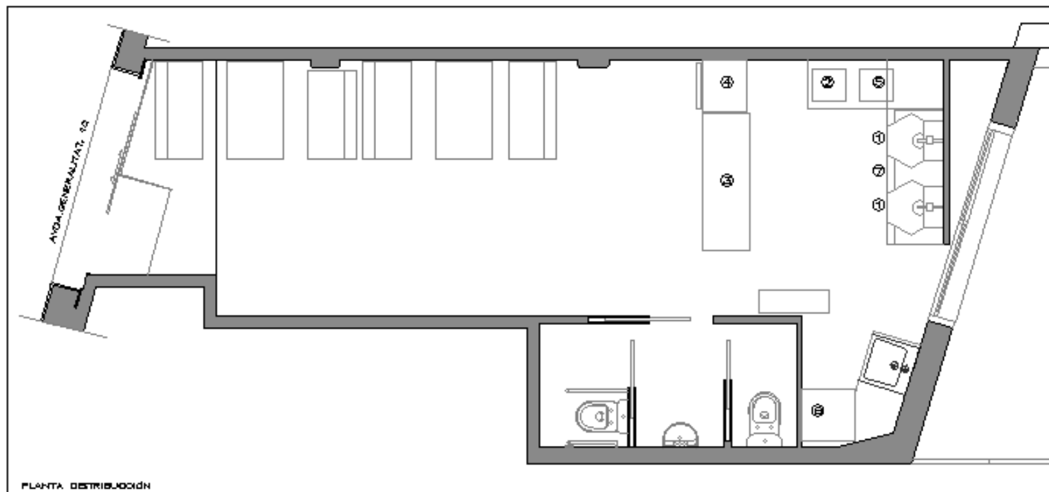
PLANTA DISTRIBUCIÓN
